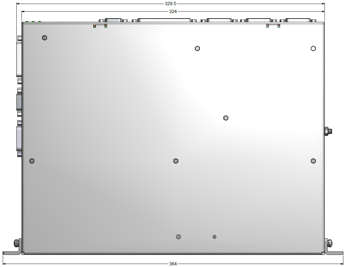
Figure 12-3. SPiiPlusCMxa Bottom
