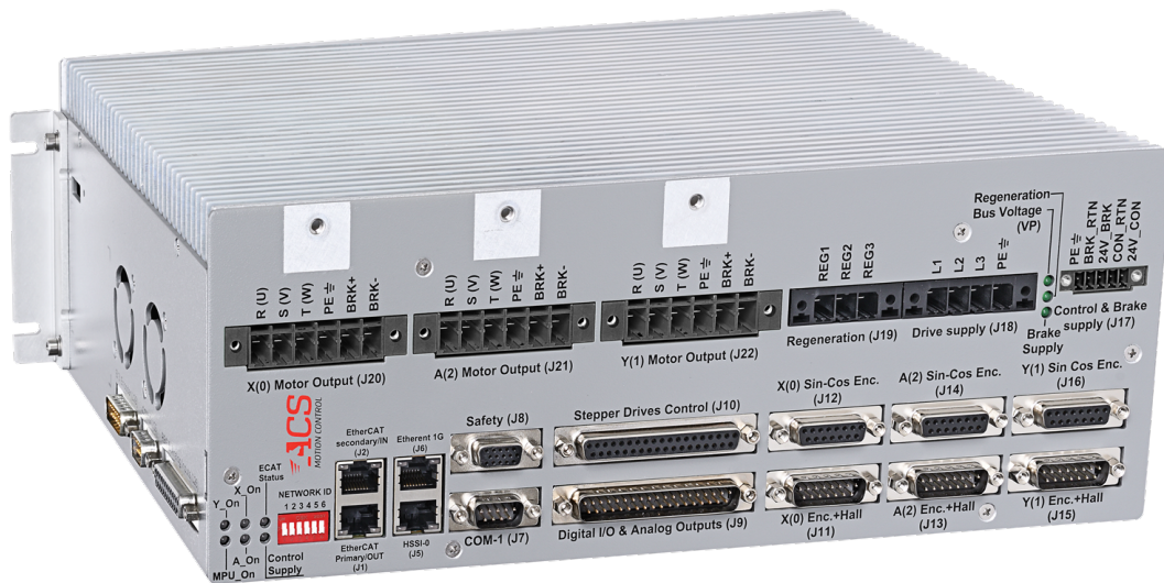
Figure 1-1. SPiiPlusCMxa
