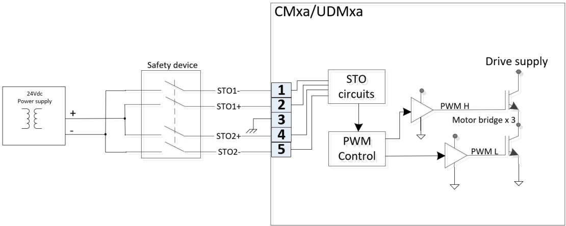
Figure 8-5. STO Inputs
