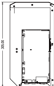
右视图
