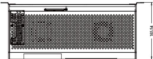
上视图
