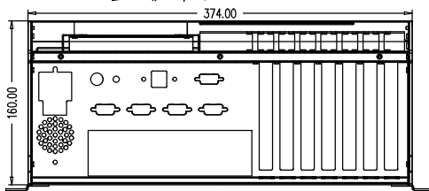
下视图
