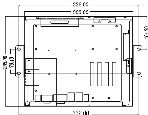
主视图
