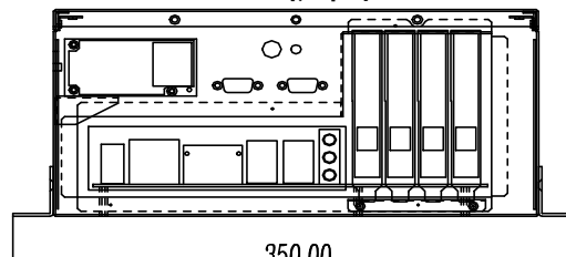
后视图
